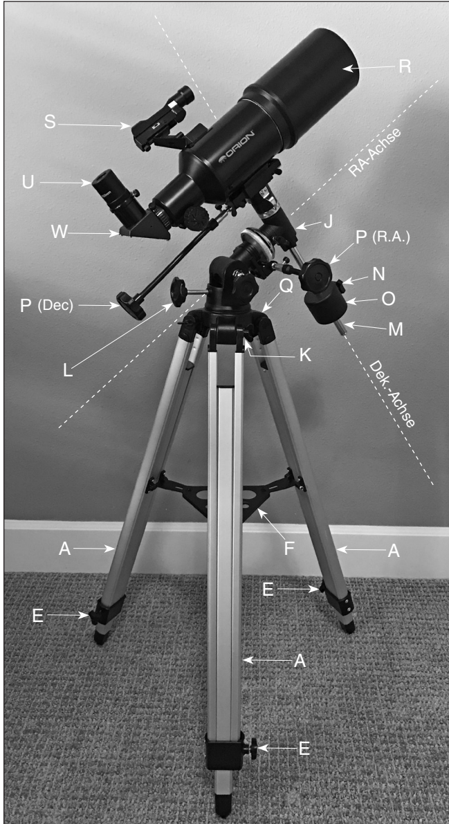
Abbildung 2. Das Observer 80ST EQ Teleskop vollständig montiert, mit Bezeichnung der wichtigsten Teile.
