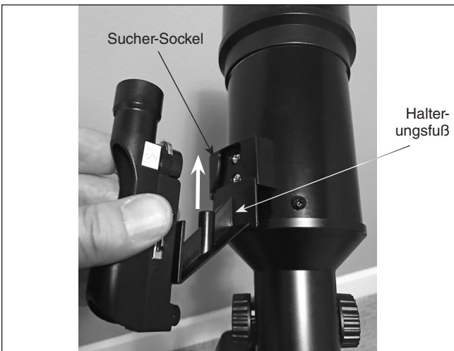
Abbildung 15. Führen Sie die Halterung des Red Dot Suchers wie gezeigt in die Basis in der Nähe des Fokussierers ein.
