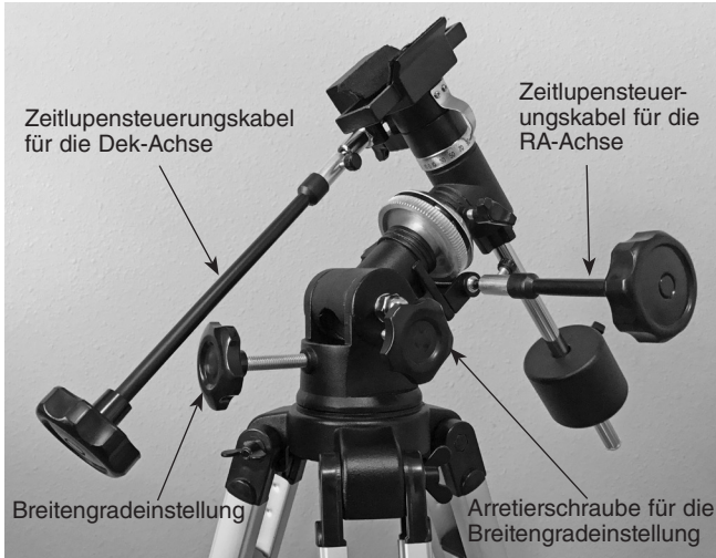
Abbildung 11. Rückansicht der parallaktischen Montierung mit den beiden angebrachten Zeitlupesteuerungskabeln.
