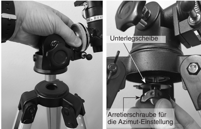
Abbildung 7. a) Installieren Sie die parallaktische Montierung auf der Stativmontageplattform, b) Sichern Sie sie dann von der Unterseite mit der Arretierschraube für die Azimuteinstellung.
