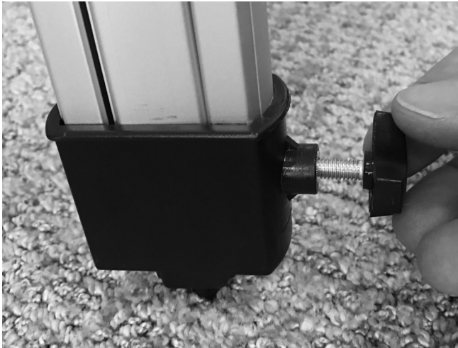
Abbildung 4. Schrauben Sie in jedes der Beine eine Rändelschraube für die Stativbeinarretierung. Seien Sie dabei vorsichtig und ziehen Sie die Schraube nicht zu fest.
