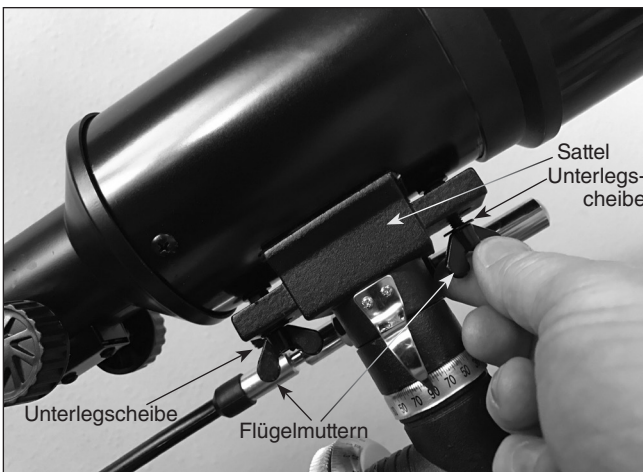
Abbildung 14. Befestigen Sie das optische Rohr mit den mitgelieferten Flügelmuttern und Unterlegscheiben an der Sattelplatte der Halterung.
