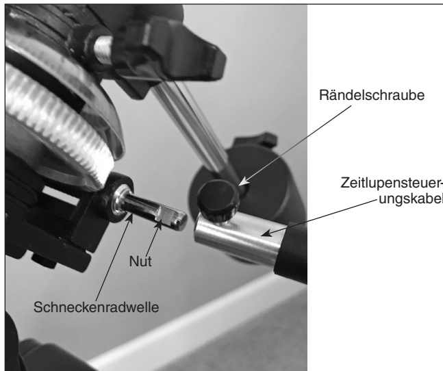
Abbildung 12. Richten Sie die Rändelschraube der Zeitlupesteuerungskabel an der Nut in der Schneckenradwelle aus und ziehen Sie sie dann fest.
