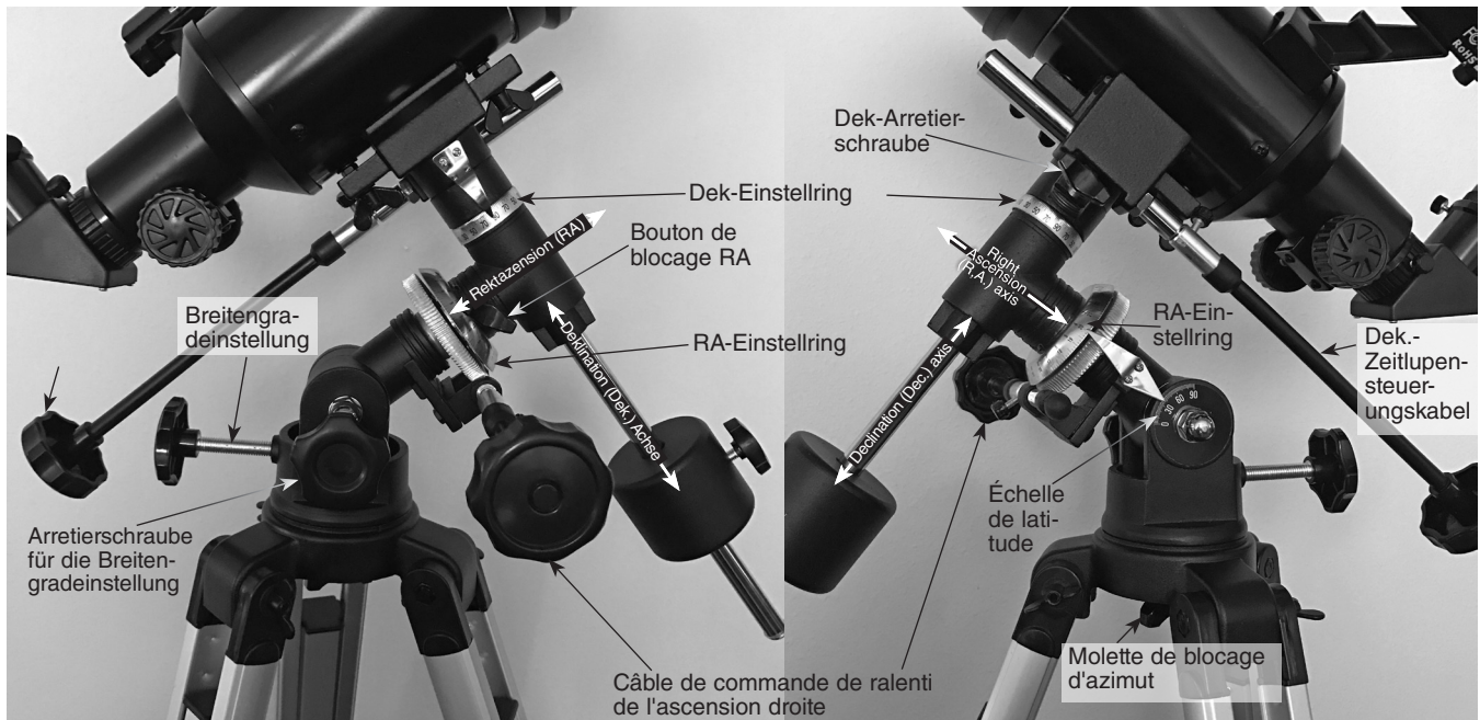
Abbildung 18. Komponenten der parallaktischen Montierung – Ansicht von beiden Seiten
