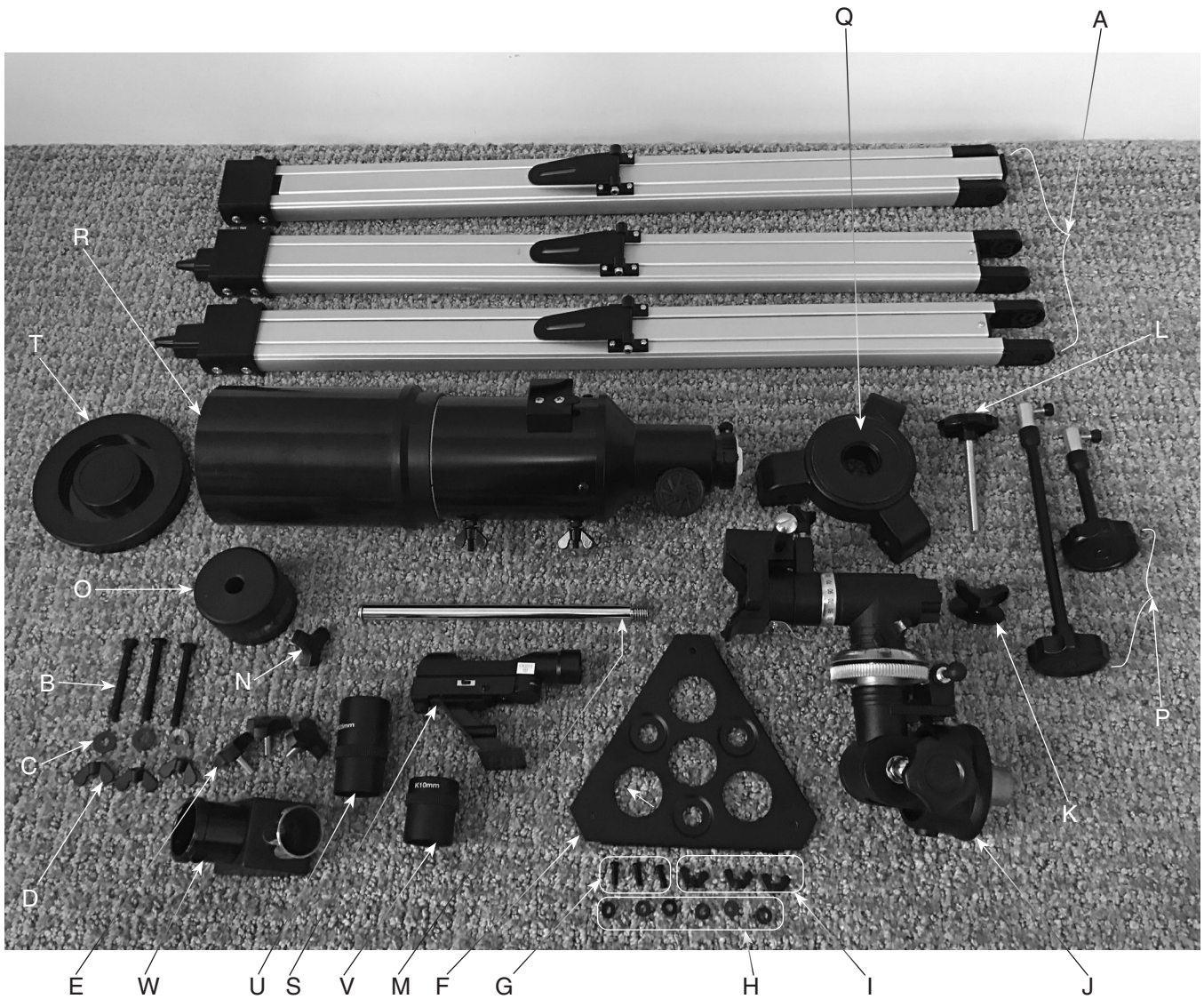
Abbildung 1. Die Teile des Observer 80ST EQ Teleskops.
